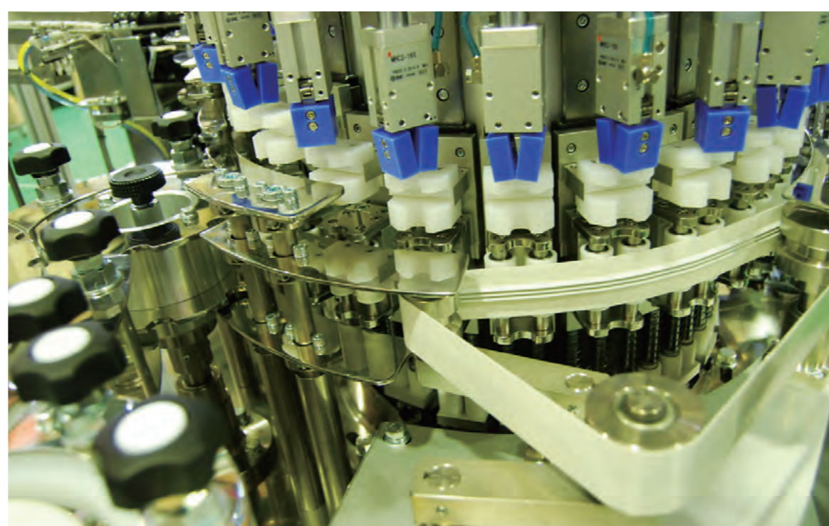
プランジャーロッド装着機構
