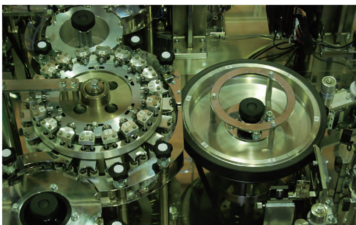
ラベル貼付け機構
