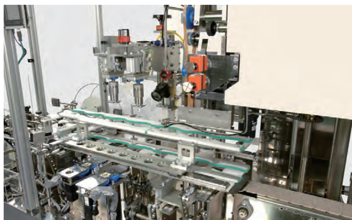
レジスター式容器方向規制装置
