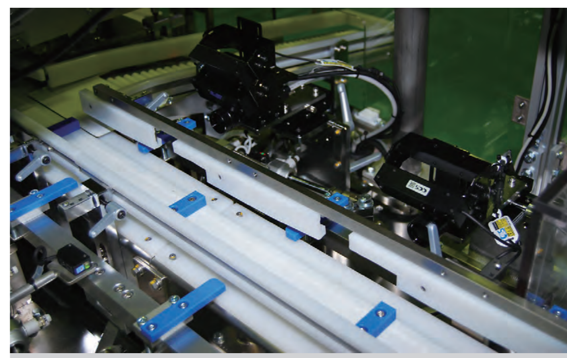
製品搬送部及び印字検査部
